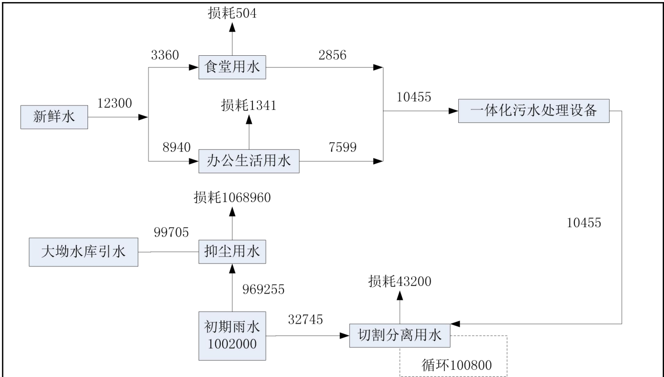
图 4-3 项目年水平衡图 单位: m³/a
