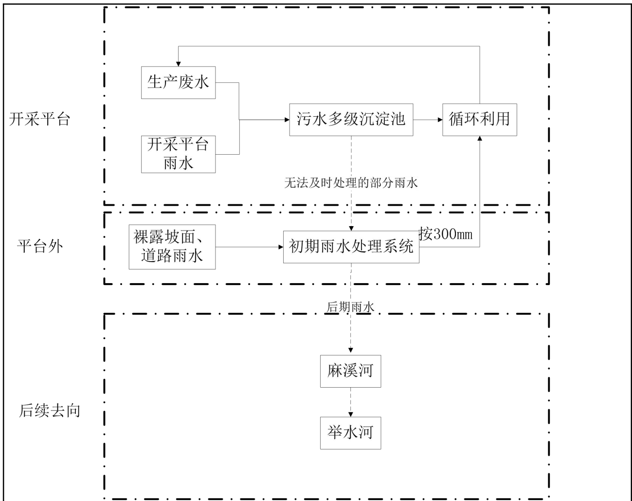
图 4-5 本项目排水流程示意图
