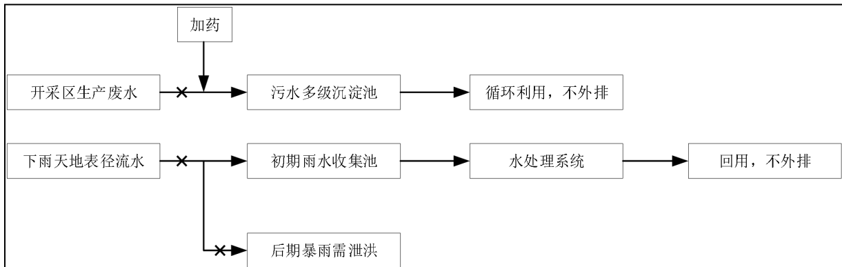
图 4-4 污、雨水收集池分流建设原则示意图
