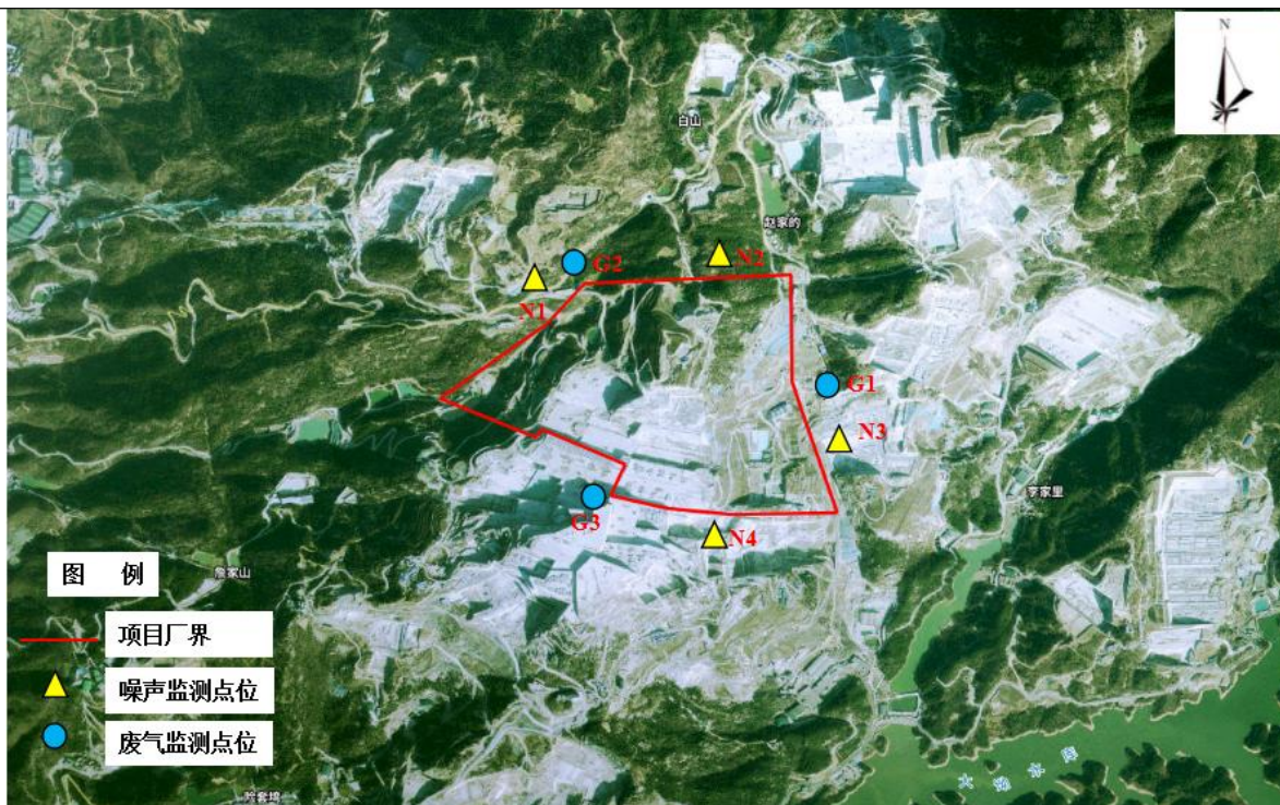
图 8-1 项目监测点位布置图
