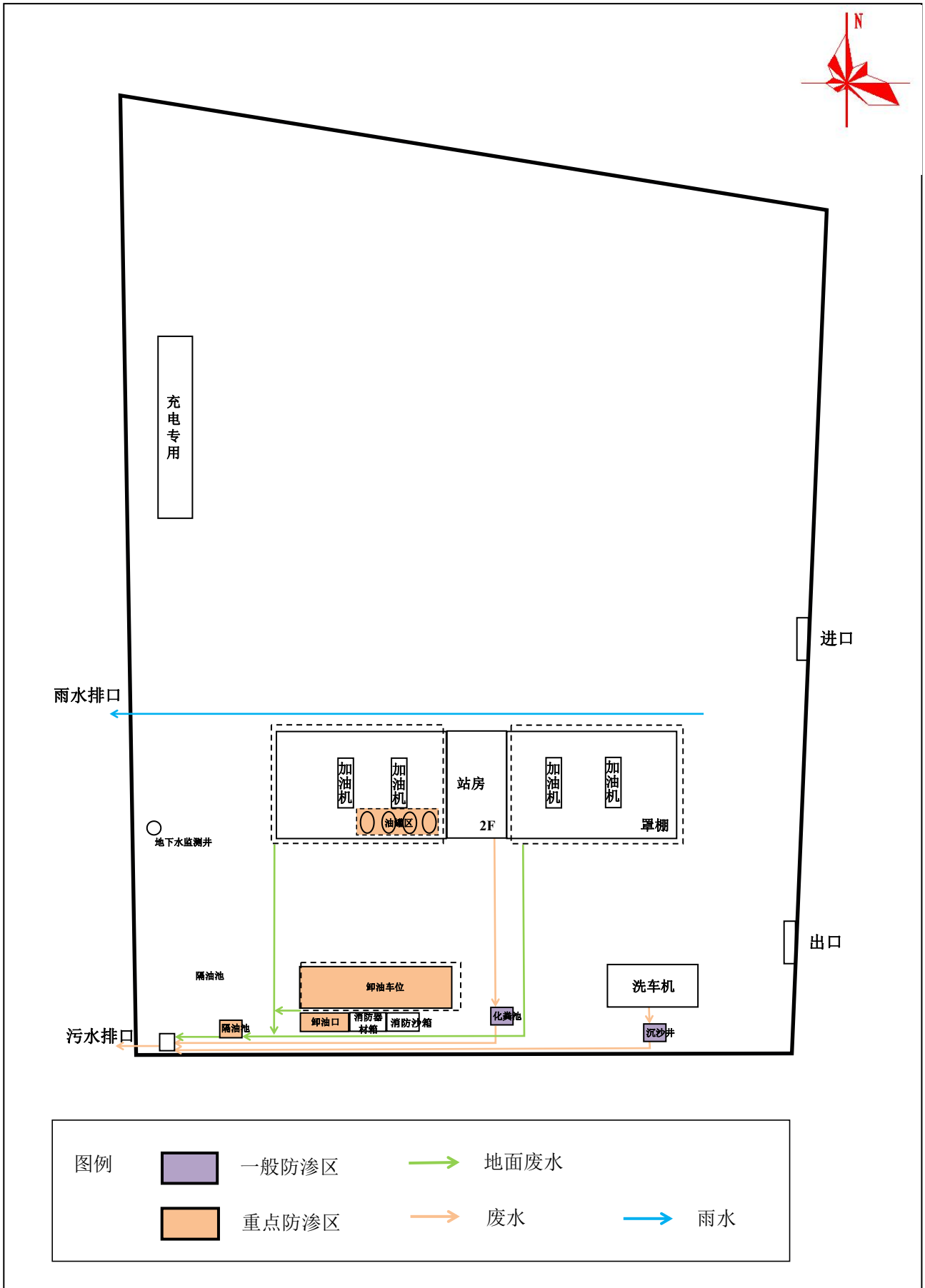
附图 3 项目平面布置及雨污管网图
