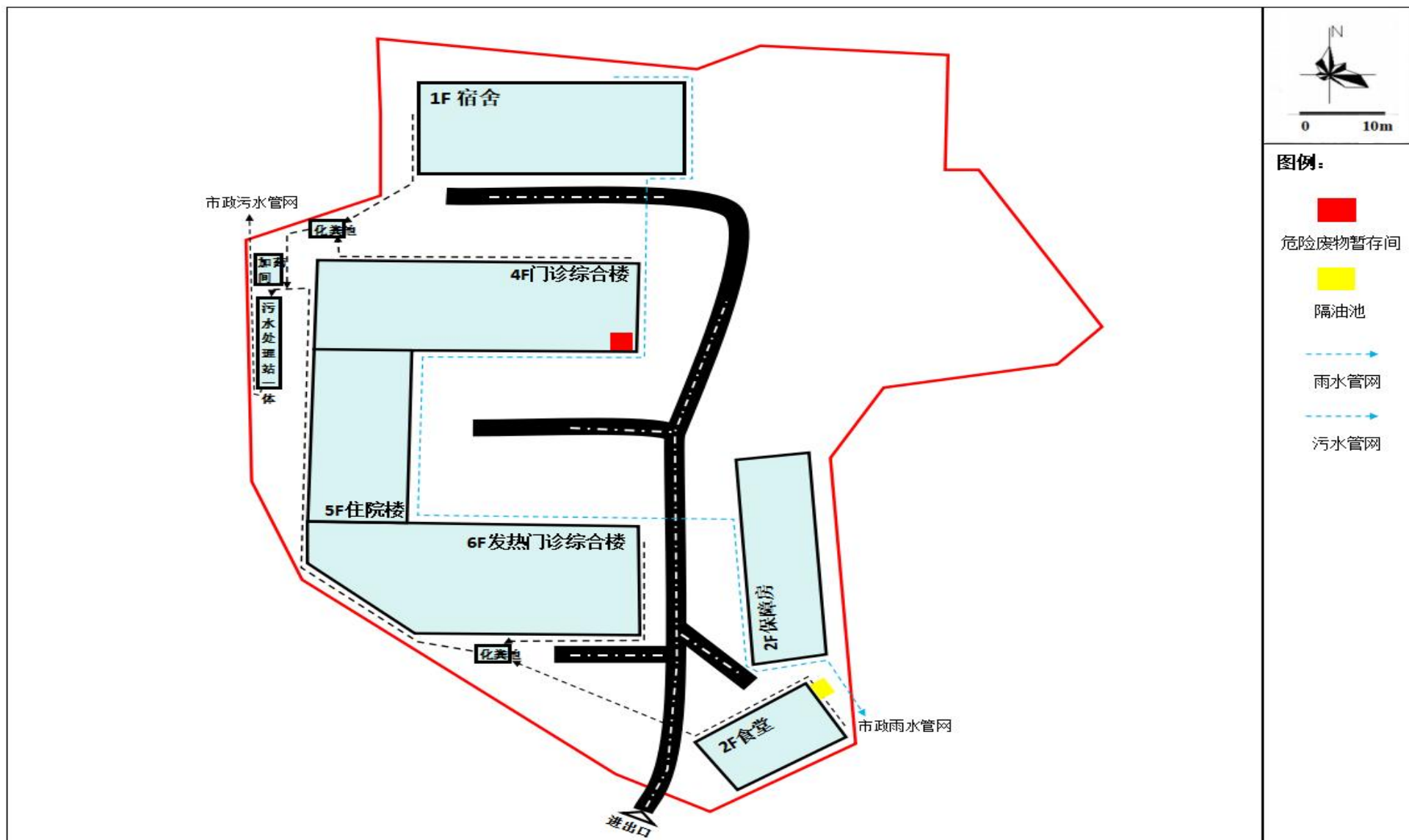
附图 4 项目总平面布置图及雨污管网图
