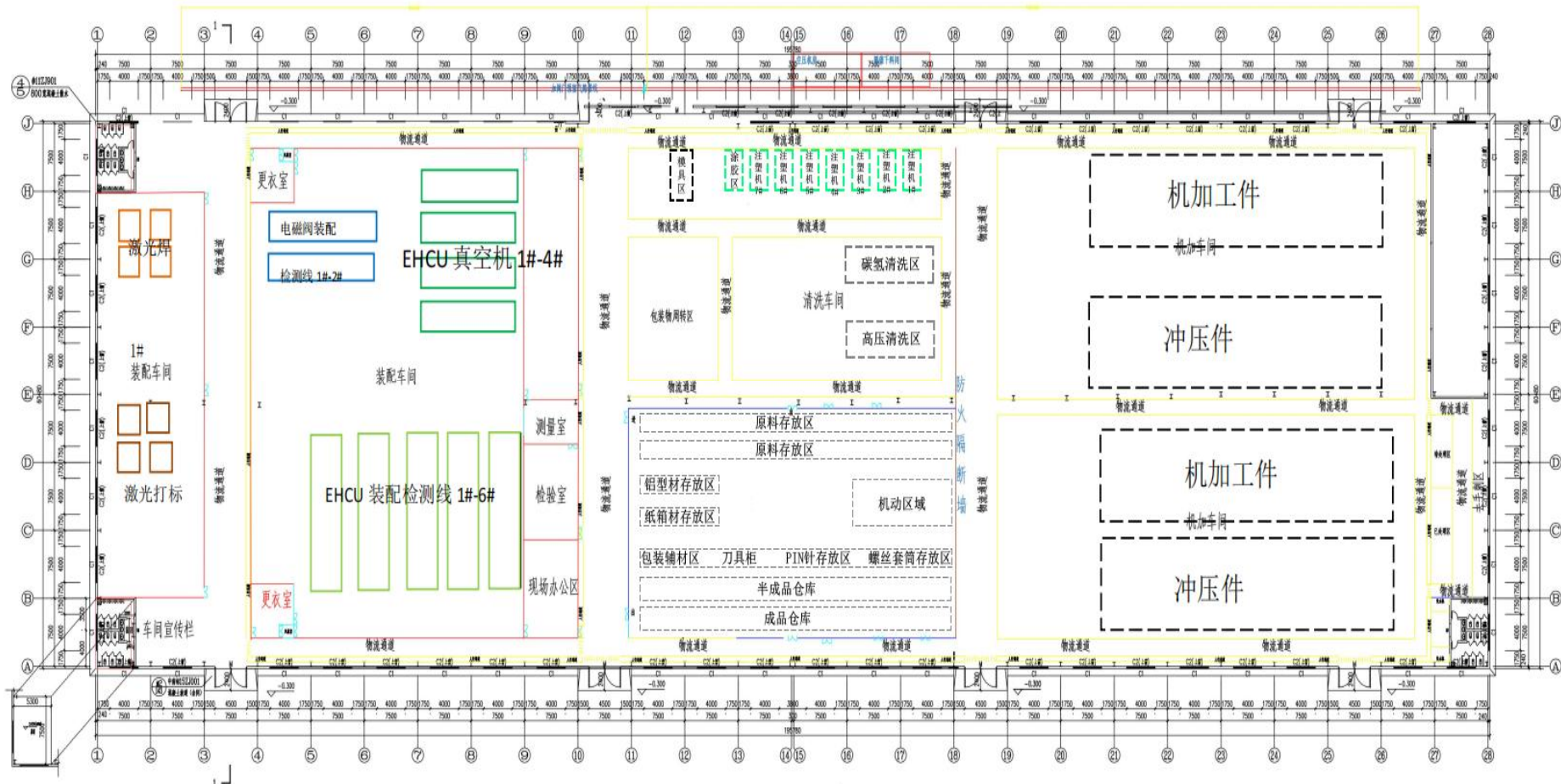
附图 4 项目生产车间平面布置图
