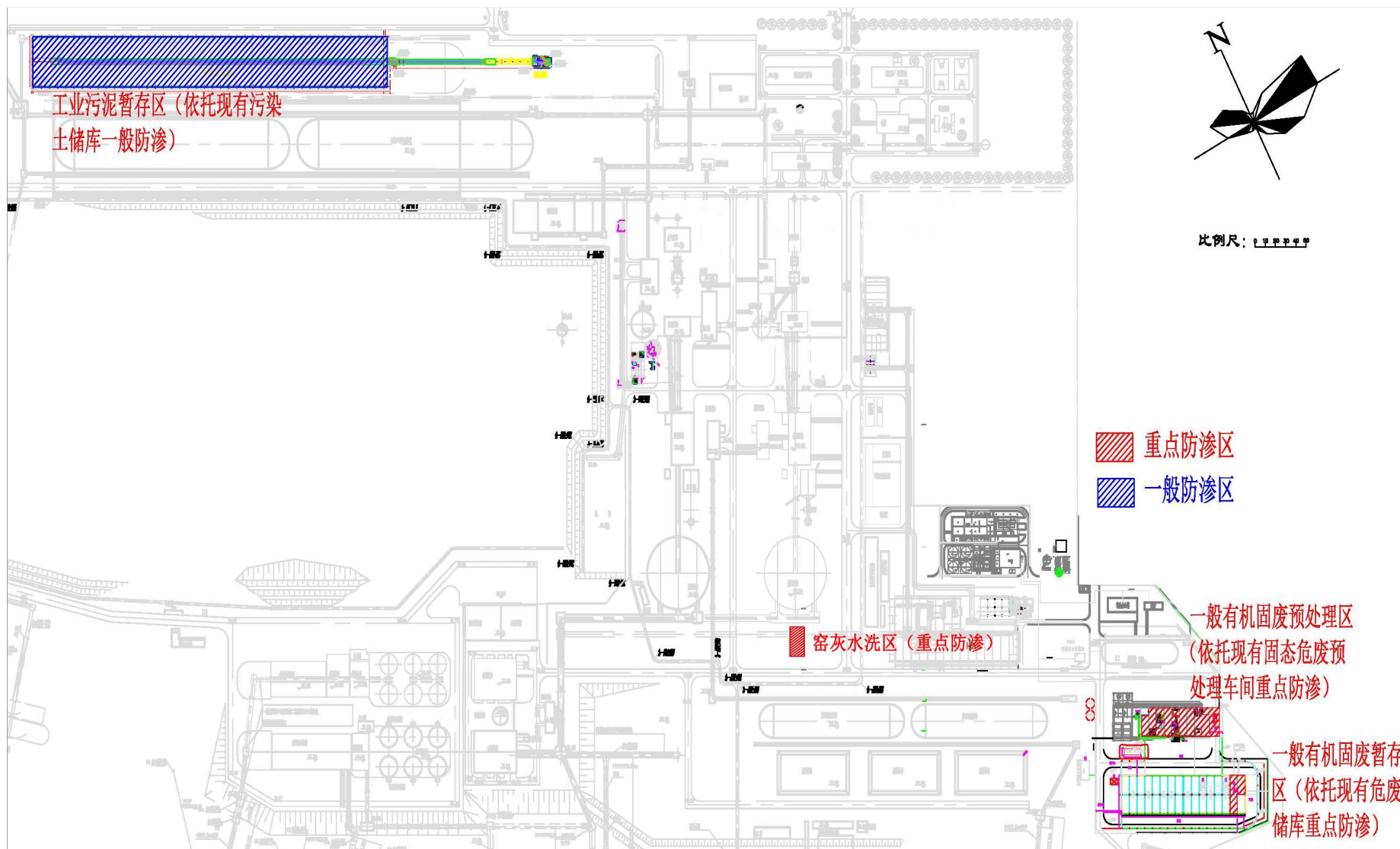
附图 6 项目分区防渗图
