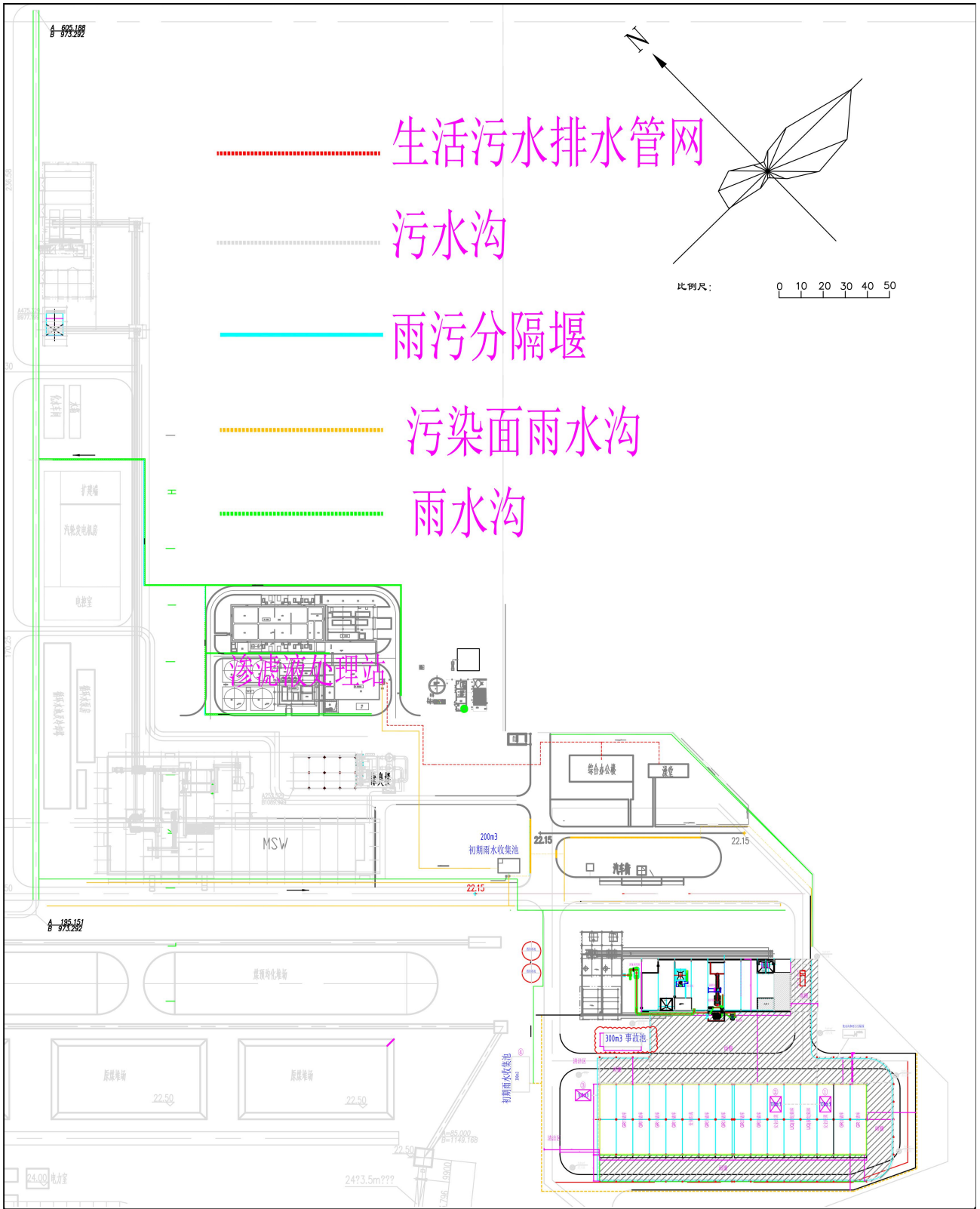
附图 4 项目（固废预处理区）雨污分流图
